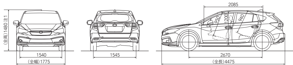
3面図(2.0i-S EyeSight) 単位:mm
